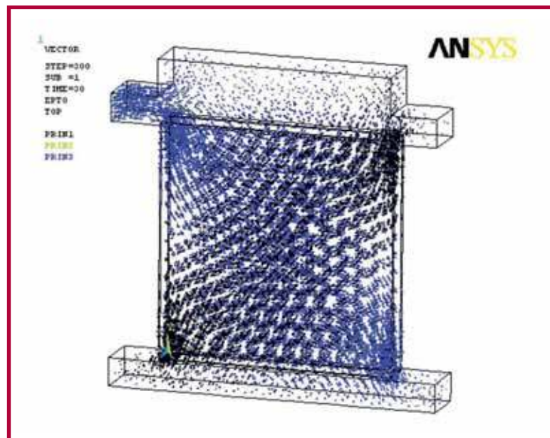
Figura 3. Simulazione numerica di test di struttura muraria rinforzata da tappezzeria antisismica (D'Appolonia) Figure 3. Numerical Simulation of seismic wallpaper composite testing (D'Appolonia)
